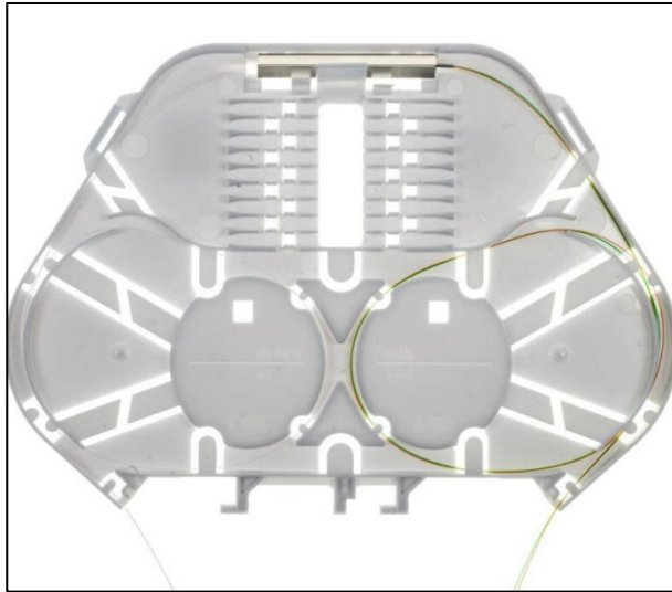
FIST-SLE (Slim Element) kassett med splitter
