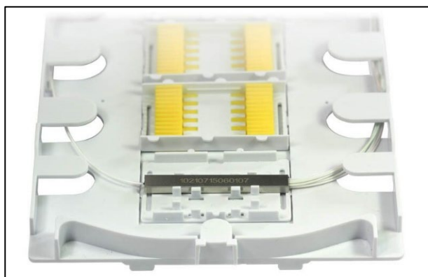
Holder med PLC splitter montert i SP-BRETT-D5-72-A
