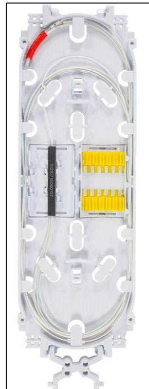
Holder med PLC splitter montert i SP-BRETT-B4-24-A
