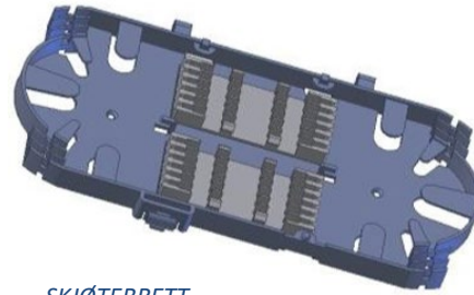
SKJØTEBRETT
