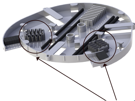
11 202 204 Multikassett för 48 singel skarvar. Med två extra hylshållare.
